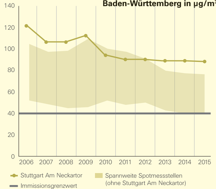
Gemessene Jahresmittelwerte des Schadstoffs Stickstoffdioxid (NO 2 ) in Baden-Württemberg in µg/m 3
